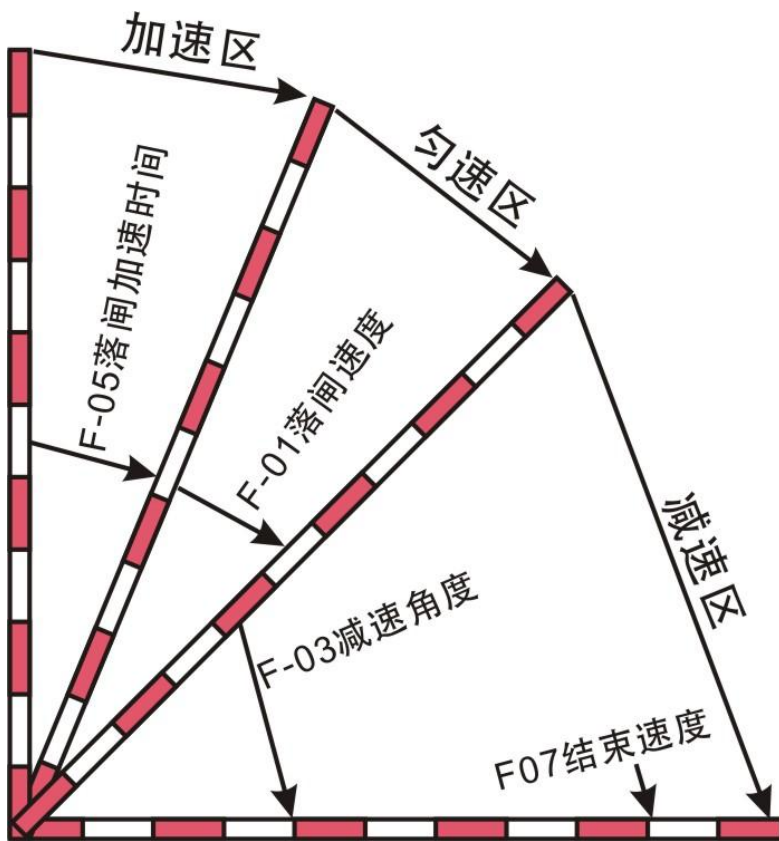
4、F-28 设置为 0 或者 F-28 设置大于等于 F-03 时的落闸示意图
